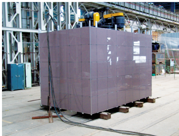
Рис.2. Общий вид испытательного стенда с конструкциями ФС «MAVent»
