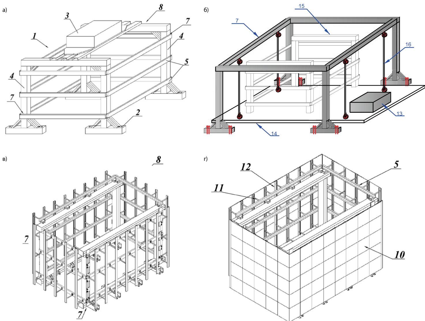
Рис.4. Схема вибростенда для динамических испытаний НВФС
