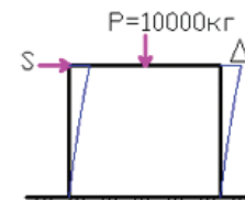
Рис.4. Схема загрузки одноэтажного фрагмента здания горизонтальной нагрузкой
