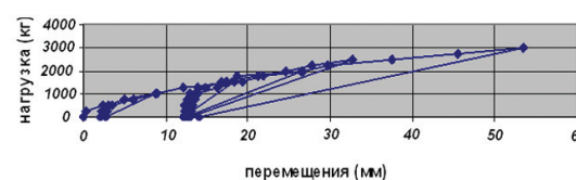
Рис.13. Зависимость горизонтальных перемещений верхних концов стоек одноэтажного фрагмента здания от горизонтальной статической нагрузки
