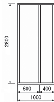
Рис.7. Эскиз панели и сечение профиля стоек
