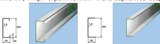
Рис.1. Стальной тонкостенный профиль
