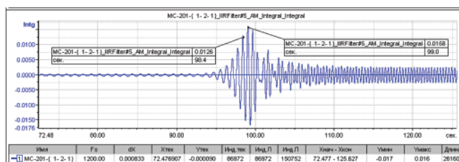
Рис.14. График изменения перемещений (м) верха стойки
