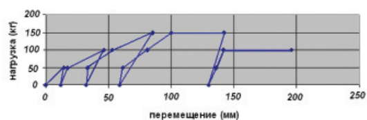
Рис.11. Зависимость горизонтальных перемещений верха стеновой панели от горизонтальной нагрузки при постоянной вертикальной нагрузке равной 0,8 Р (6000 кг)
