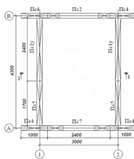
Рис.8. Схема фрагмента здания
