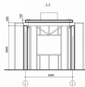
Рис.8. Схема фрагмента здания
