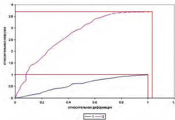
Рис.13. График изменения физико-механических свойств образцов кирпичной кладки: 1 - эталонный образец; 2 - образец, усиленный с использованием СНО.
