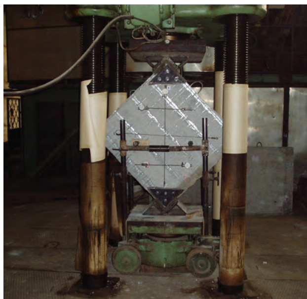
Рис.9. Железобетонный образец, изготовленный с использованием СНО
